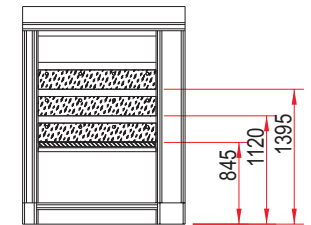
3 étages
